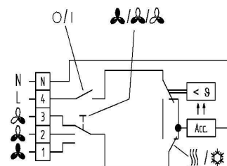
KLR-E 7015 kapcsolási rajza:
